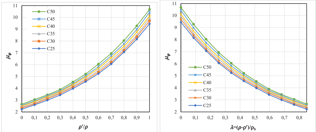
Şekil 2.3. Basınç/çekme donatısı oranının ve beton basınç dayanımının moment ve eğrilik davranışı üzerindeki etkisi
