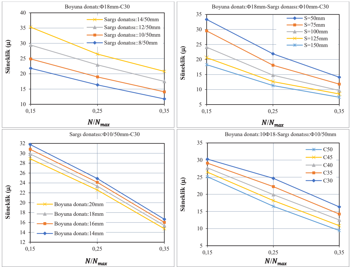
Şekil 4.4. Betonarme perde duvar kesitlerinde farklı tasarım parametrelerinin eğrilik sünekliliği üzerindeki etkisinin karşılaştırmalı gösterimi
