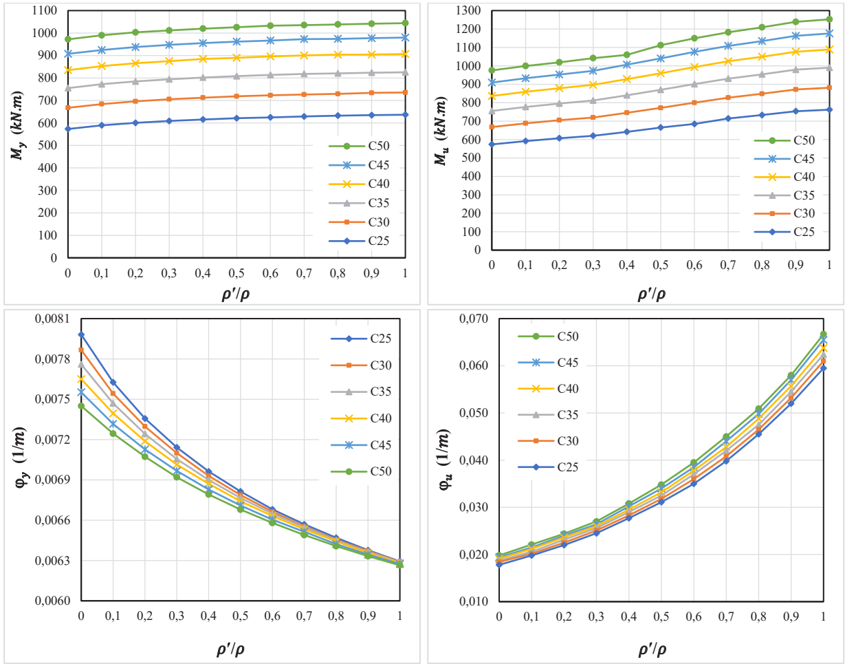
Şekil 2.3. Basınç/çekme donatısı oranının ve beton basınç dayanımının moment ve eğrilik davranışı üzerindeki etkisi
