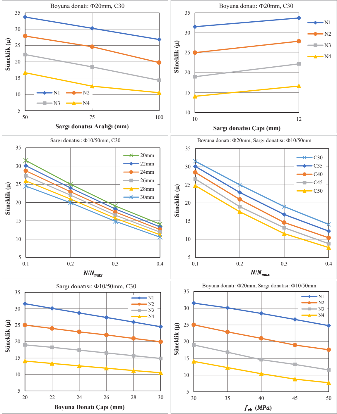
Şekil 3.7. 400 mm × 600 mm dikdörtgen en-kesitli kolonlar için farklı tasarım parametrelerinin eğrilik sünekliği üzerindeki etkisi
