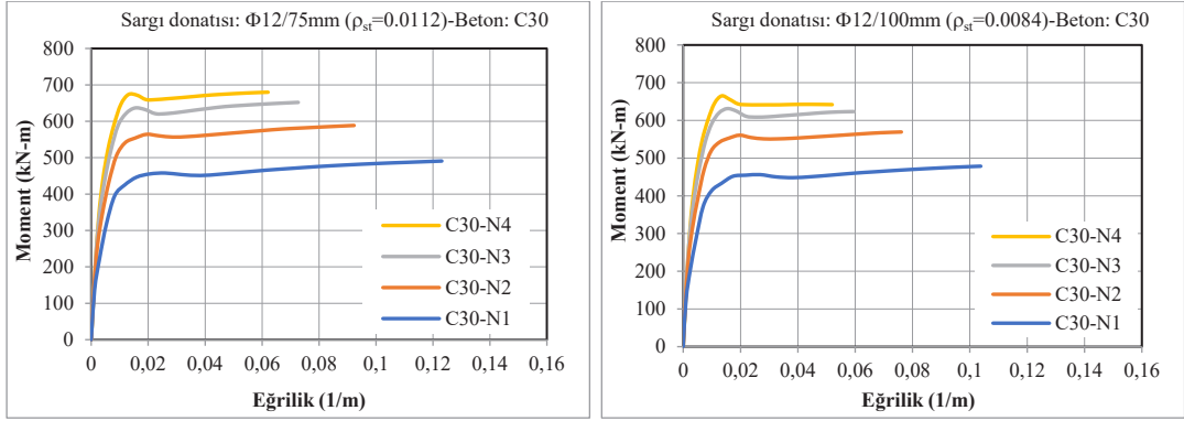
a) Farklı sargı donatısı oranı (boyuna donatı: 8\Phi 20 - beton: C30)
