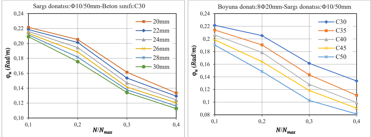
Şekil 3.3. 500 mm × 500 mm kare kesitli kolonlar için farklı tasarım parametrelerinin moment ve eğrilik değerleri üzerindeki etkisi
