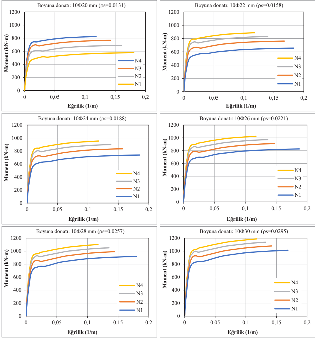
b) Farklı boyuna donatı oranı (sargı donatısı: \Phi 10/50 mm - beton: C30)
