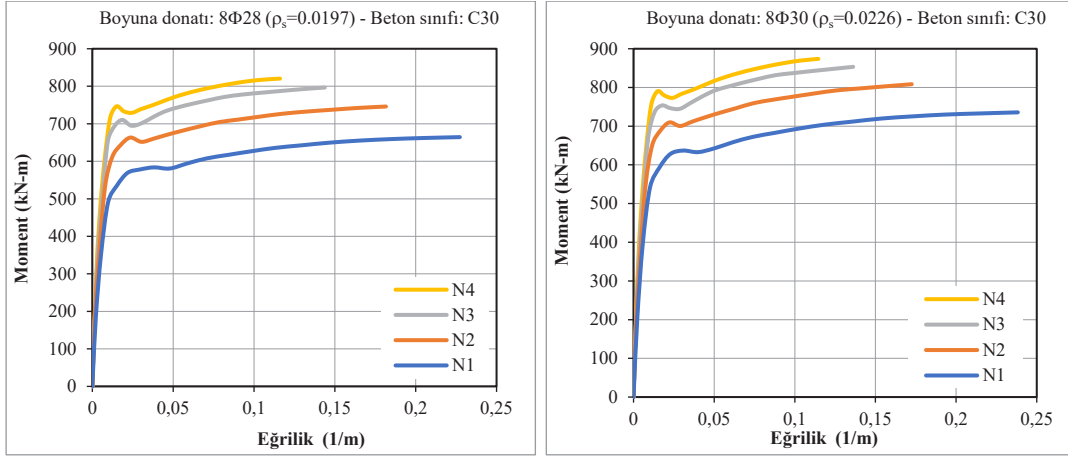
b) Farklı boyuna donatı oranı (sargı donatısı: Φ10/50 mm - beton sınıfı: C30)
