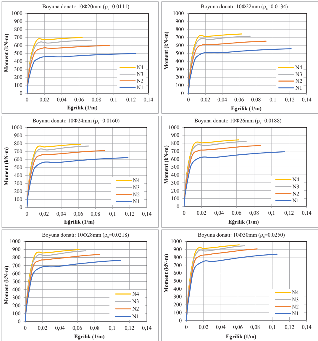
b) Farklı boyuna donatı oranı (sargı donatısı: \Phi 10/50\text{mm} - beton: C30)
