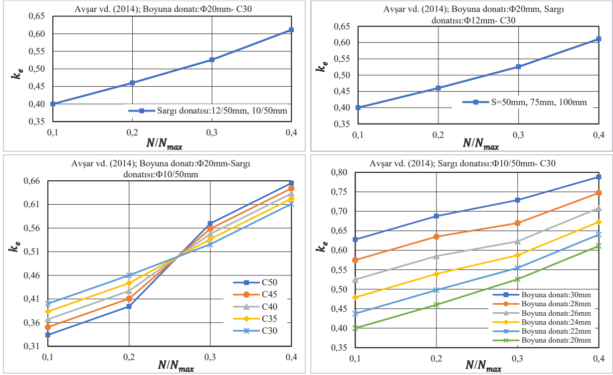
Şekil 3.26. 400 mm × 600 mm dikdörtgen enkesitli kolonun Avşar vd. (2014) yaklaşımından elde edilen etkin eğilme rijitliği katsayısının farklı parametrelere bağlı değişimi
