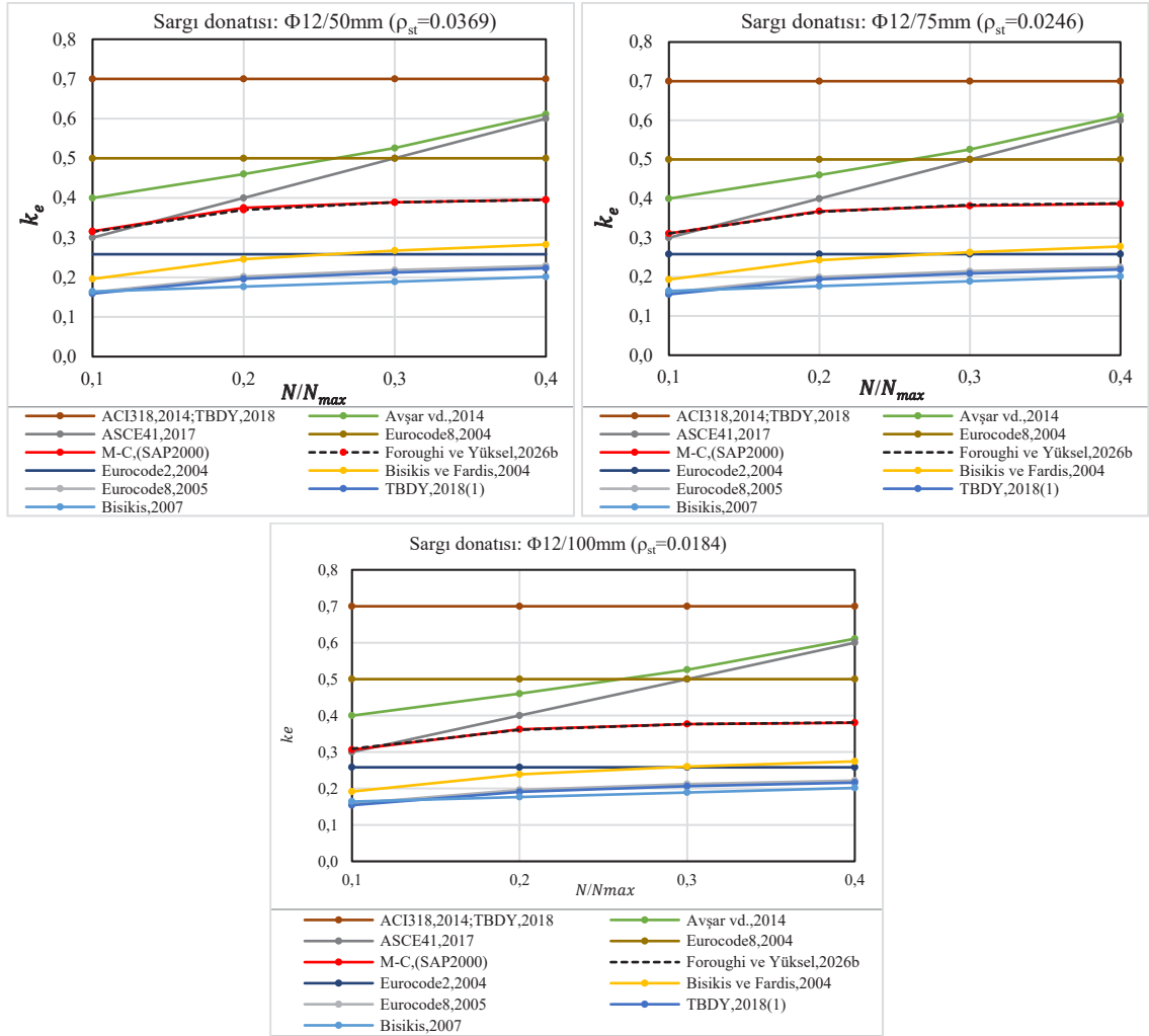
Şekil 3.35. 500 mm \times 500 mm kare enkesitli kolonların farklı tasarım parametrelere göre k_e - N/N_{max} ilişkileri
