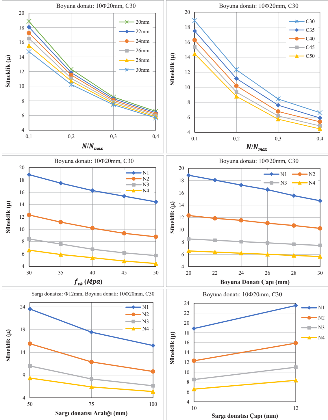
Şekil 3.10. 600 mm dairesel enkesitli kolonlar için farklı tasarım parametrelerinin eğrilik sünekliği üzerindeki etkisi
