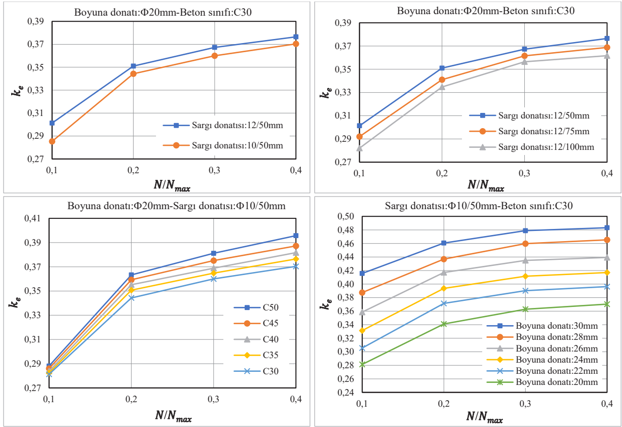
Şekil 3.11. 500 mm x 500 mm kare enkesitli kolonun farklı parametrelerine göre moment-eğrilik ilişkilerinden elde edilen k_e ilişkileri.
