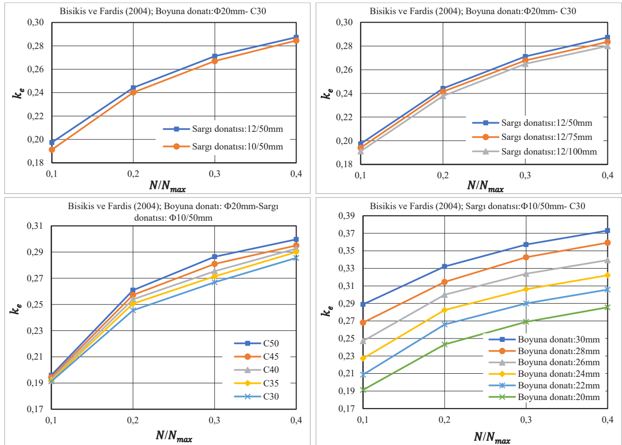
Şekil 3.21. 500 mm × 500 mm kare enkesitli kolonun Bisikinis ve Fardis (2004) yaklaşımından elde edilen etkin eğilme rijitliği katsayısının farklı parametrelere bağlı değişimi
