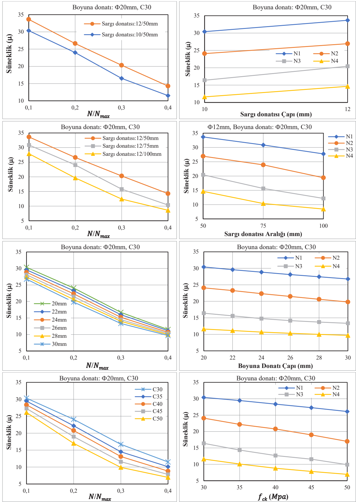
Şekil 3.4. 500 mm × 500 mm kare enkesitli kolonlar için farklı tasarım parametrelerinin eğrilik sünekliği üzerindeki etkisi
