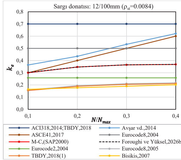
a) Farklı sargı donatısı oranına göre k_e - N/N_{max} grafikleri (boyuna donatı: \Phi 20 mm- beton sınıfı: C30)
