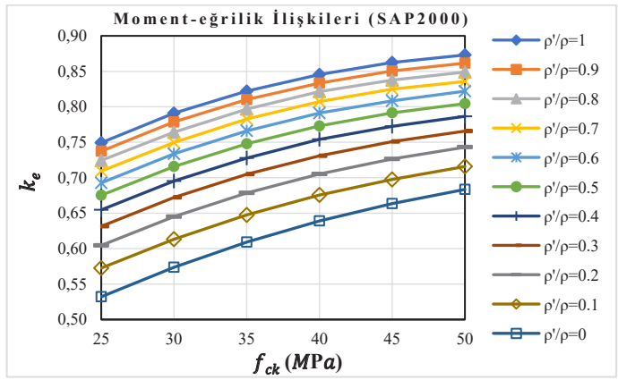
Şekil 2.5. Betonarme kirişlerde moment-eğrilik ilişkilerinden elde edilen etkin eğilme rijitliği katsayılarına \rho'/\rho oranı ve f_{ck} parametrelerinin etkisi
