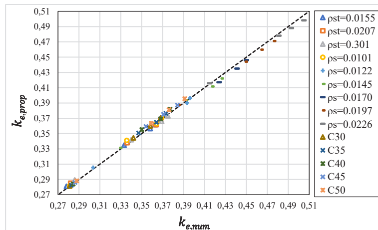
Şekil 3.32. 500 mm x 500 mm kare enkesitli betonarme kolonların k_{e,prop} - k_{e,num} ilişkilerinin karşılaştırılması
