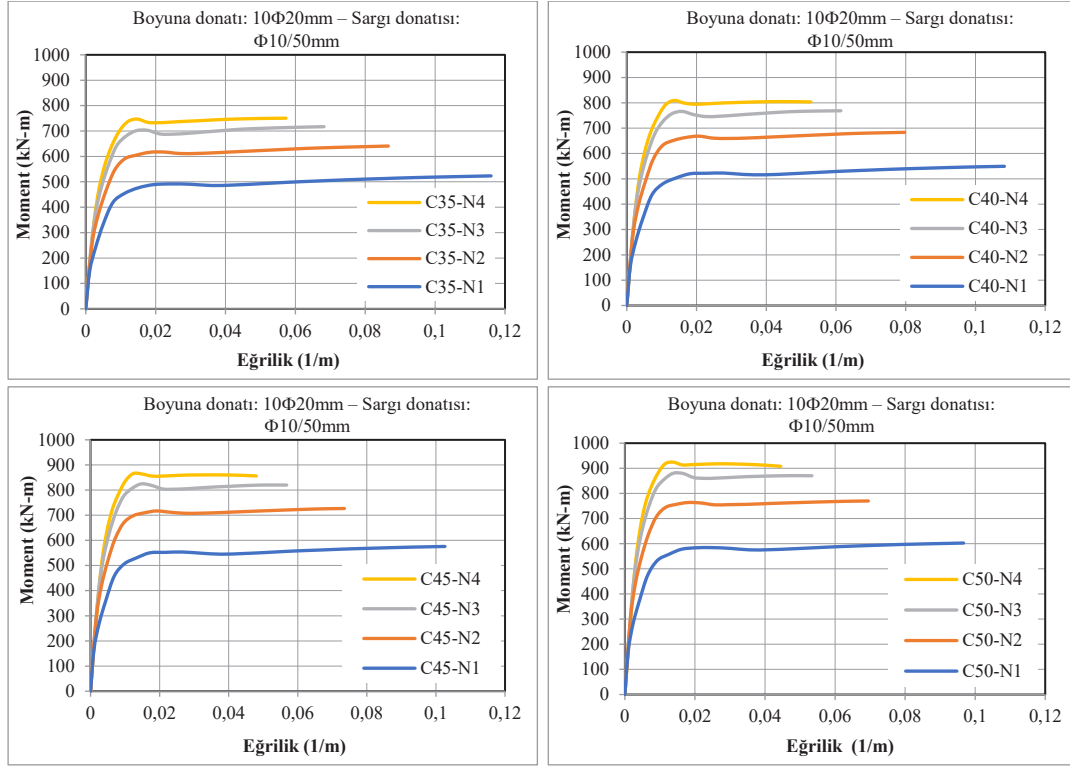
c) Farklı beton basınç dayanımı (boyuna donatı: 10Φ20 mm - sargı donatısı: Φ10/50 mm) Şekil 3.8. Farklı tasarım parametreleri için 600 mm dairesel enkesitli kolonların moment-eğrilik ilişkilerinin karşılaştırılması.
