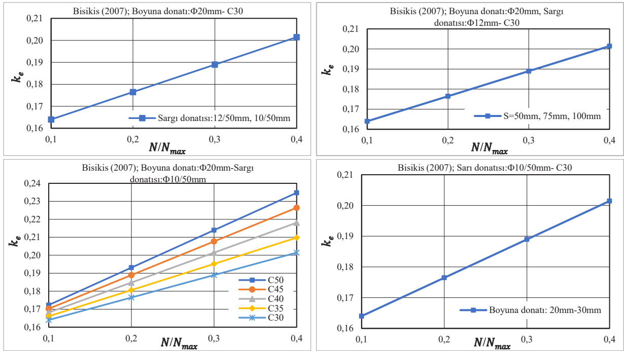
Şekil 3.25. 400 mm x 600 mm dikdörtgen enkesitli kolonun Bisikis (2007) yaklaşımından elde edilen etkin eğilme rijitliği katsayısının farklı parametrelere bağlı değişimi
