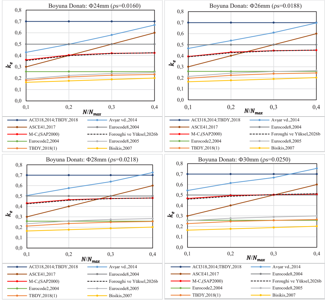
b) Farklı boyuna donatı oranına göre k_e - N/N_{max} grafikleri (sargı donatısı: \Phi 10/50 mm- beton sınıfı: C30)
