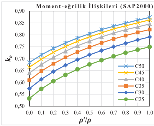
Şekil 2.5. Betonarme kirişlerde moment-eğrilik ilişkilerinden elde edilen etkin eğilme rijitliği katsayılarına \rho'/\rho oranı ve f_{ck} parametrelerinin etkisi
