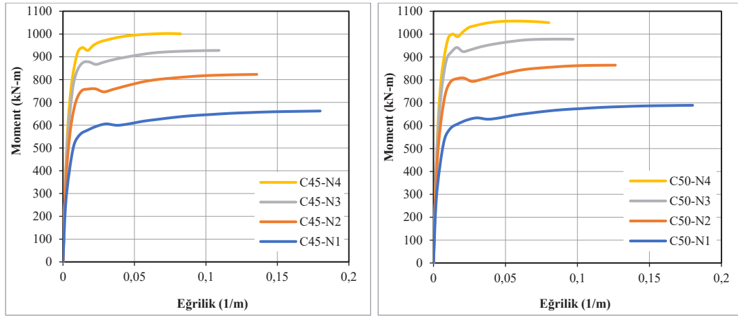
Şekil 3.5. Farklı tasarım parametreleri için 400 mm×600 mm dikdörtgen en-kesitli kolonların moment-eğrilik ilişkilerinin karşılaştırılması.
