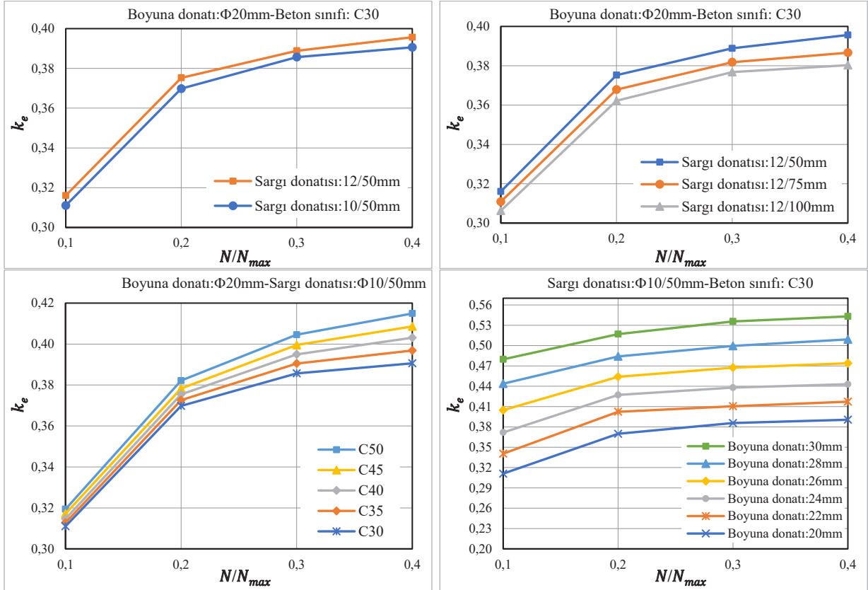
Şekil 3.12. 400 mm×600 mm dikdörtgen enkesitli kolonun farklı parametrelerine göre moment-egrilik ilişkilerinden elde edilen k_e ilişkileri.
