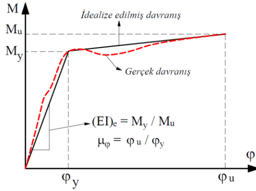
Şekil 1.3. Betonarme kesitlerde moment-eğrilik ilişkisinin idealize edilmiş gösterimi ile eğrilik sünekliliği ve etkin kesit rijitliği kavramlarının şematik tanımı.
