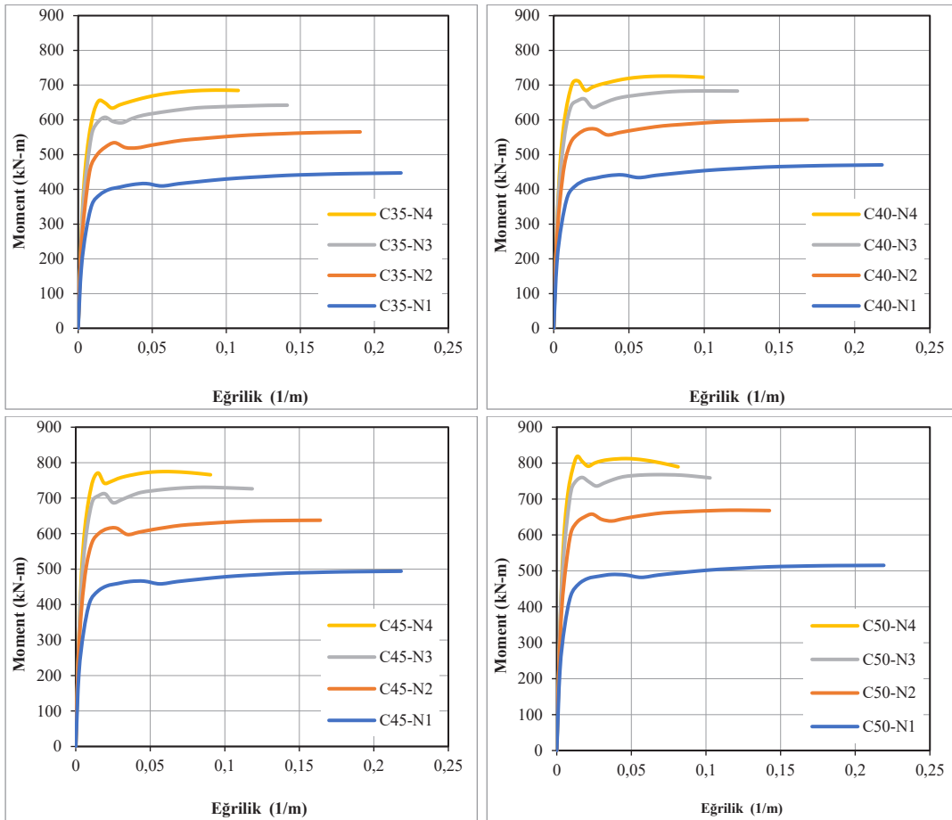
c) Farklı beton basınç dayanımı (boyuna donatı: 8Φ20 mm - sargı donatısı: Φ10/50 mm)
