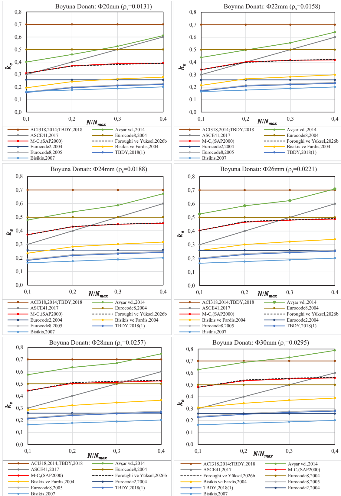
b) Farklı boyuna donatı oranına göre k_e - N/N_{max} grafikleri (sargı donatısı: \Phi 10/50 mm- beton sınıfı: C30)
