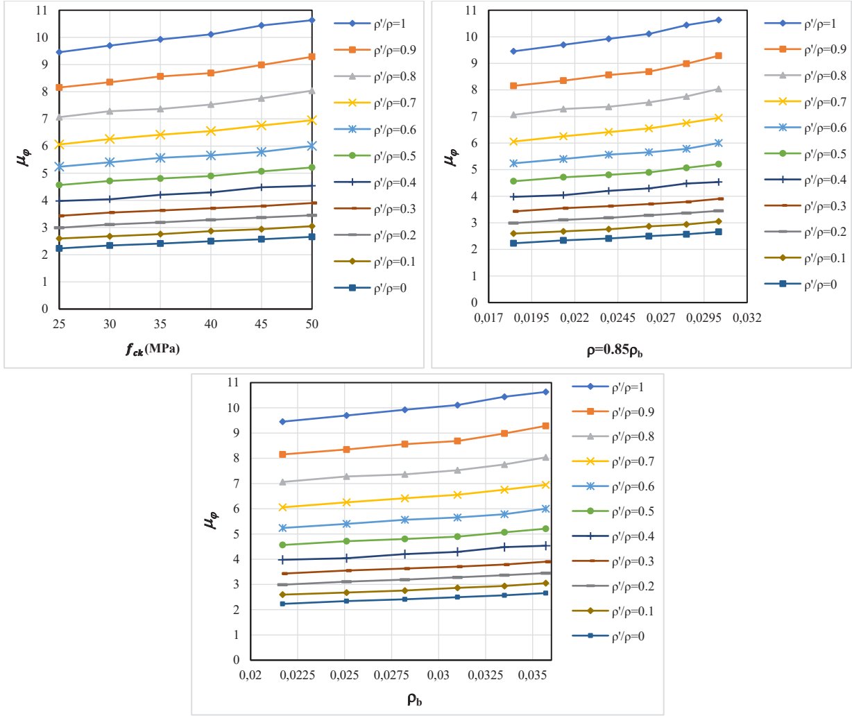
Şekil 2.4. Farklı tasarım parametrelerinin betonarme kiriş elemanların eğrilik sünekliği üzerindeki etkisi
