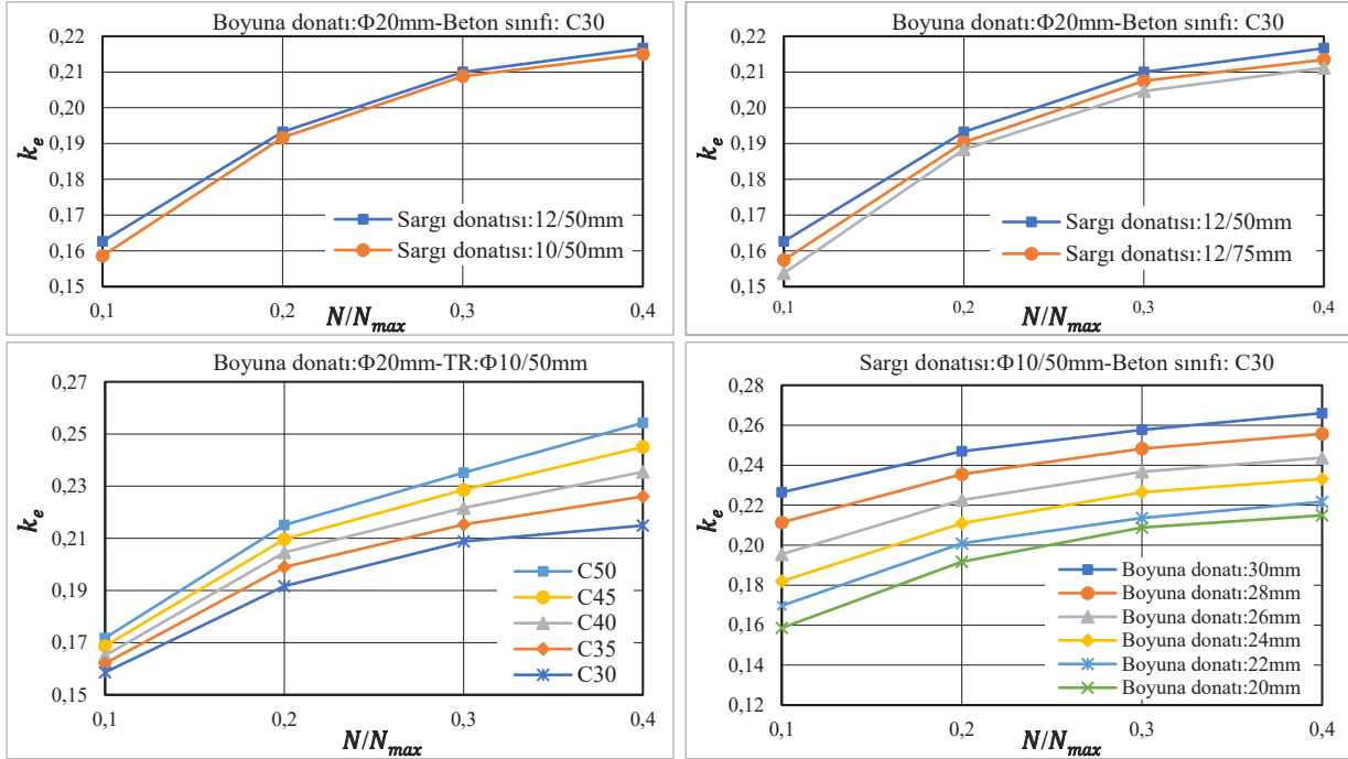
Şekil 3.17. 600 mm dairesel enkesitli kolonun TBDY (2018)'e göre yığılı plastik davranış yaklaşımı kapsamında elde edilen k_e ilişkileri
